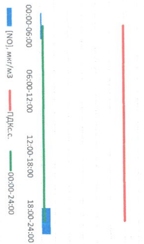
NO, мкг/м 3
